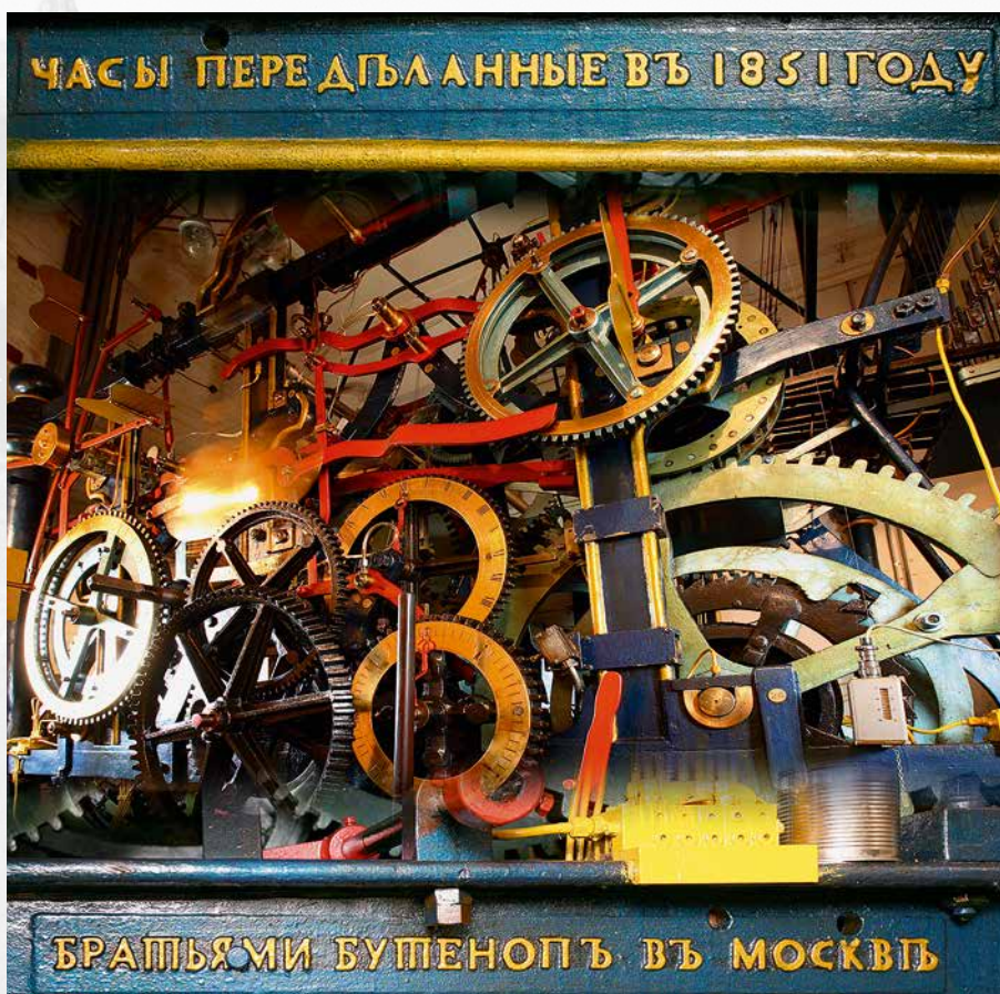
Механизм кремлёвских часов, реконструированный братьями Бутеноп в 1851-1852 гг
