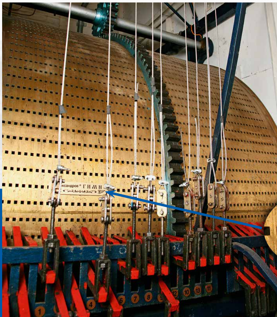
Музыкальный механизм Кремлевских курантов и главный музыкальный барабан, воспроизводящий мелодию Государственного Гимна Российской Федерации
